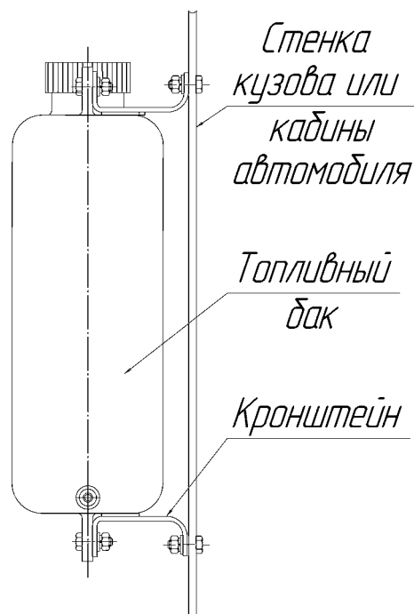
Рис. 6- Установка топливного бака на автомобиль.
