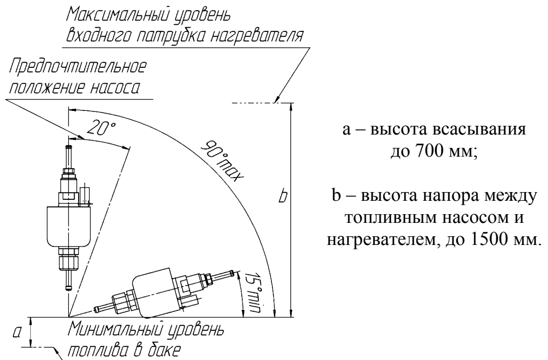
Рис. 8- Допустимое монтажное положение топливного насоса
